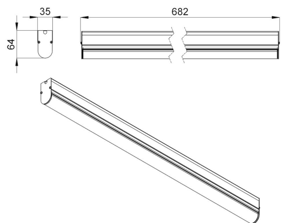
Габаритный чертеж
