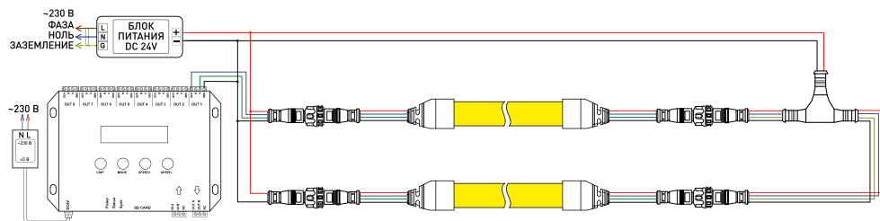
Рис. 1. Схема подключения питания с обеих сторон неона и использованием одного источника напряжения
