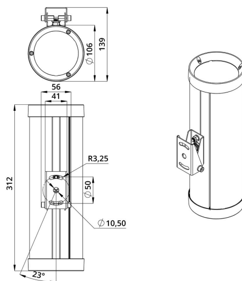
Габаритный чертеж
