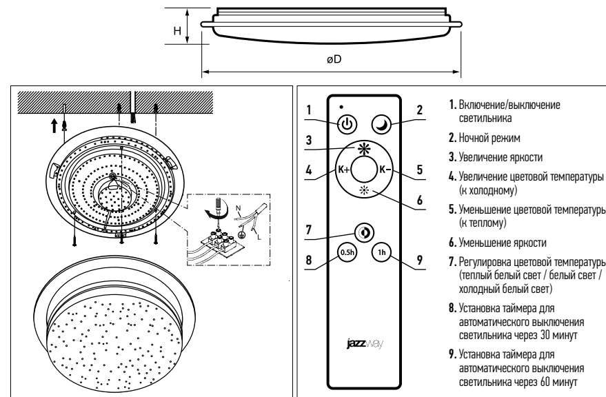
Рис 1. Светильник PPB
